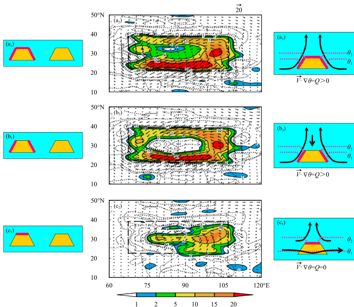
图1 \sigma=0.991 坐标面上风速(矢量, 单位: m/s)和垂直速度( -\omega )(色阶, 单位: \times 10^2 Pa/s)的差异分布(a. 全地形感热影响, b. 地形斜坡感热影响, c. 地形平台感热影响; a 1 —c 1 , 试验设计; a 2 —c 2 , 大气运动特征; a 3 —c 3 , 相关机制示意; 橘黄填色代表地形, 加粗红短线表示给定了地表感热加热, 虚矩形表示给定梯形山脉的底部; 改自 Wu, et al, 2007)
