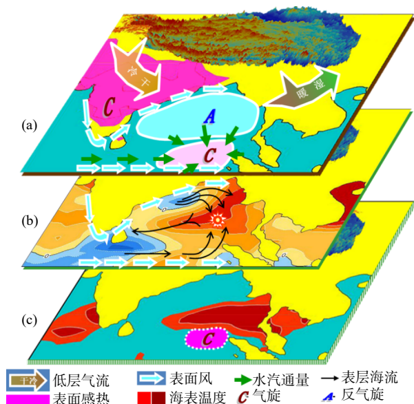
图3 春季在青藏高原强迫和南亚海陆热力对比共同作用下孟加拉湾暖池形成和季风暴发涡旋激发示意 (a. 青藏高原大气环流调节和南亚海陆热对比, b. 表层洋流和海温变化, c. 孟加拉湾暖池的形成和亚洲夏季季风暴发涡旋; Wu, et al, 2012a)
